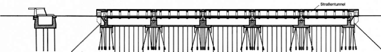
LÄNGSSCHNITT
